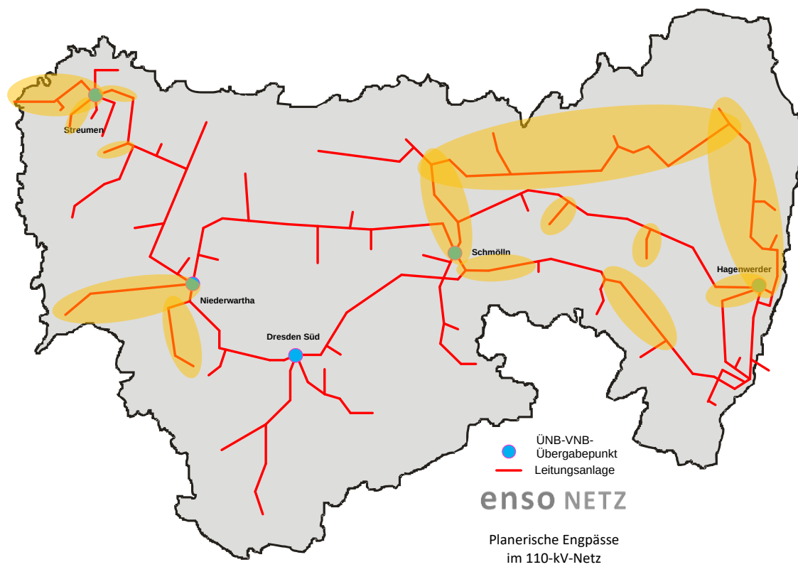
Abbildung 6: Engpässe im Hochspannungsnetz der ENSO NETZ
