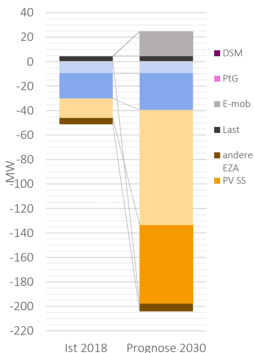
Leistungen im Lastfall Schwachlast/ starke Erzeugung
