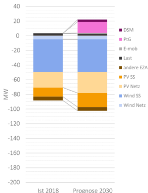
Leistungen im Lastfall Schwachlast/ starke Erzeugung
