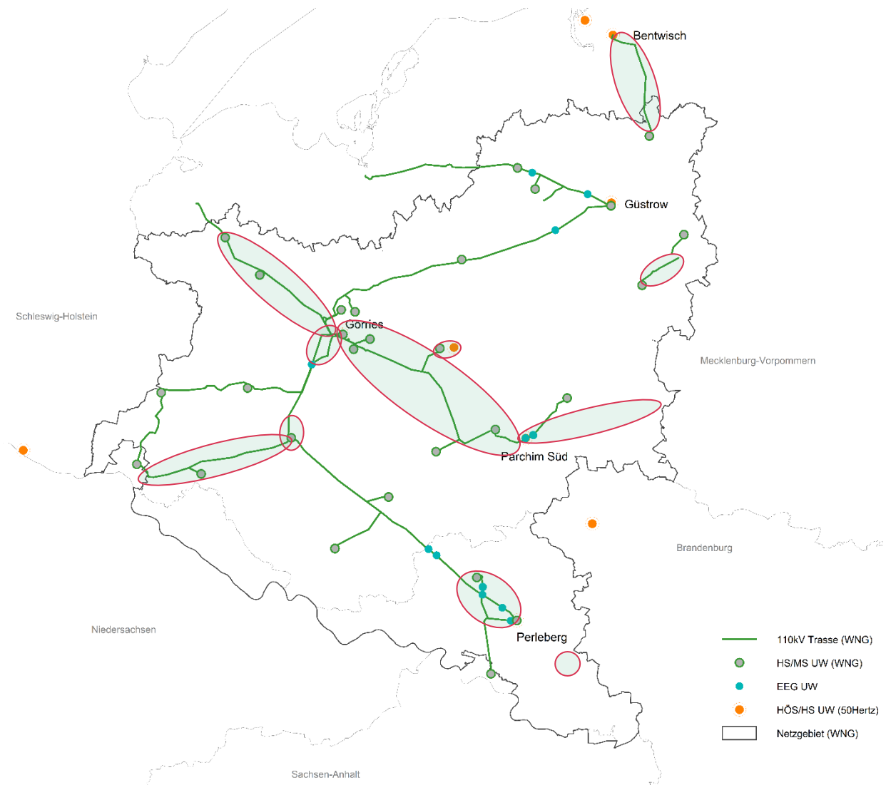
Abbildung 16: Leitungsbaumaßnahmen im HS-Netz der WEMAG Netz GmbH
