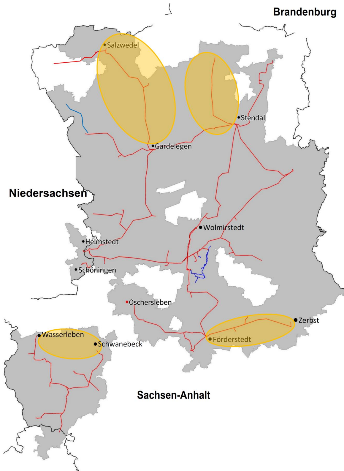
Abbildung 4: Engpässe im Hochspannungsnetz der Avacon Netz (nur Regelzone 50Hertz)
