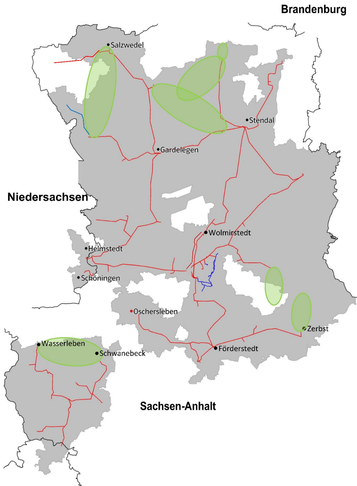
Abbildung 11: Leitungsbaumaßnahmen im HS-Netz der Avacon Netz
