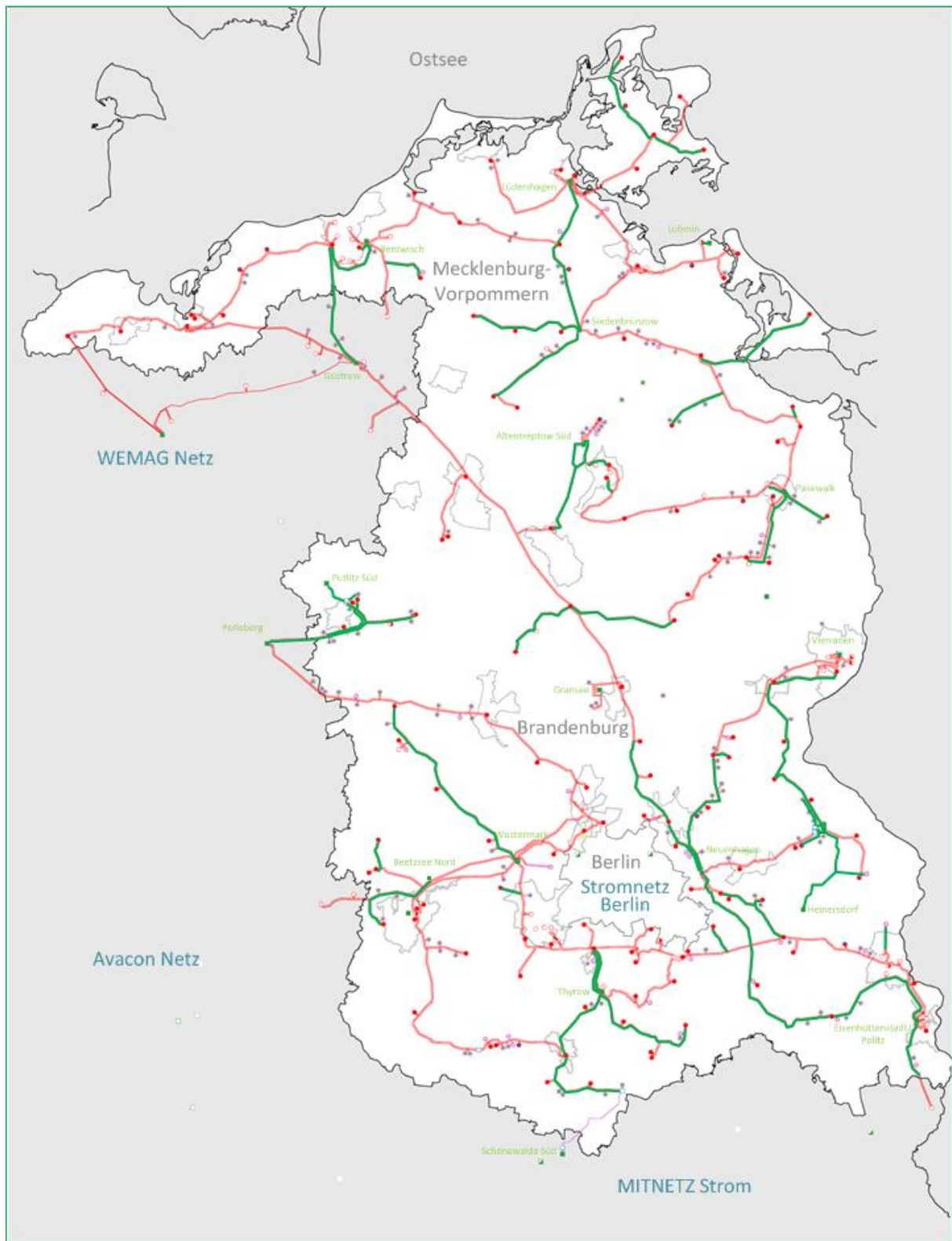
Abbildung 12: Leitungsbaumaßnahmen im HS-Netz der E.DIS Netz
