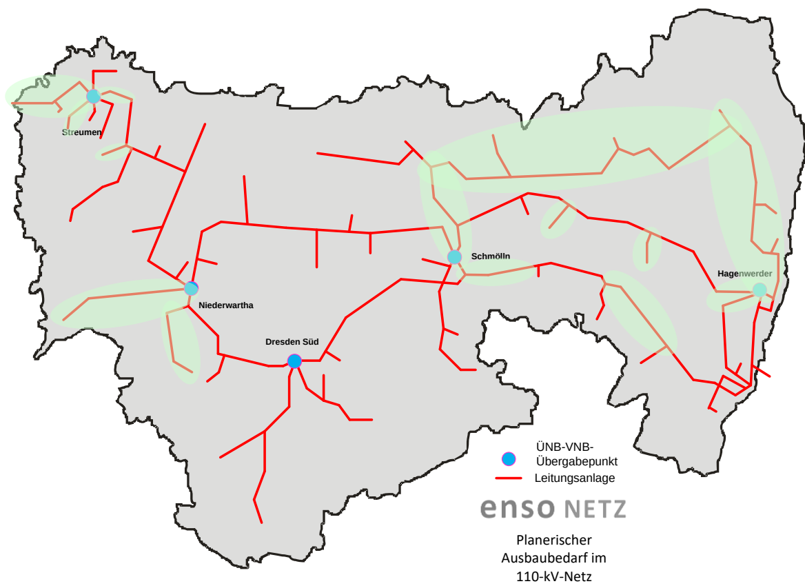
Abbildung 13: Leitungsbaumaßnahmen im HS-Netz der ENSO NETZ
