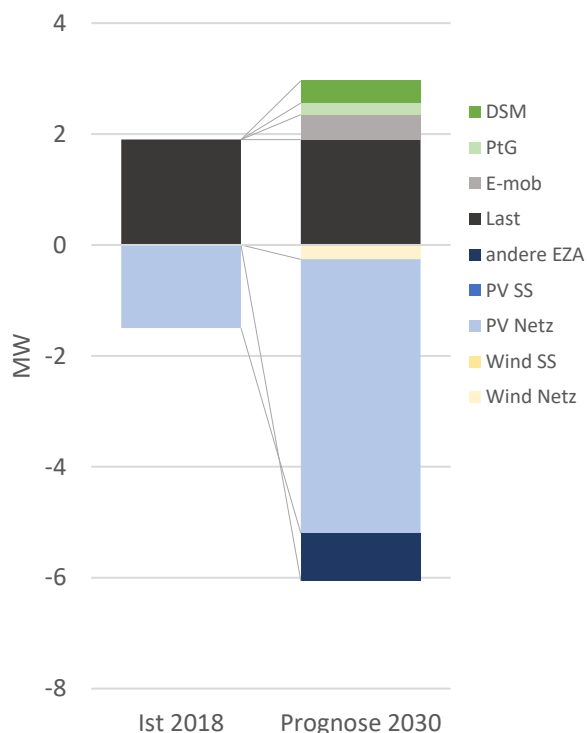
Leistungen im Lastfall Schwachlast/ starke Erzeugung
