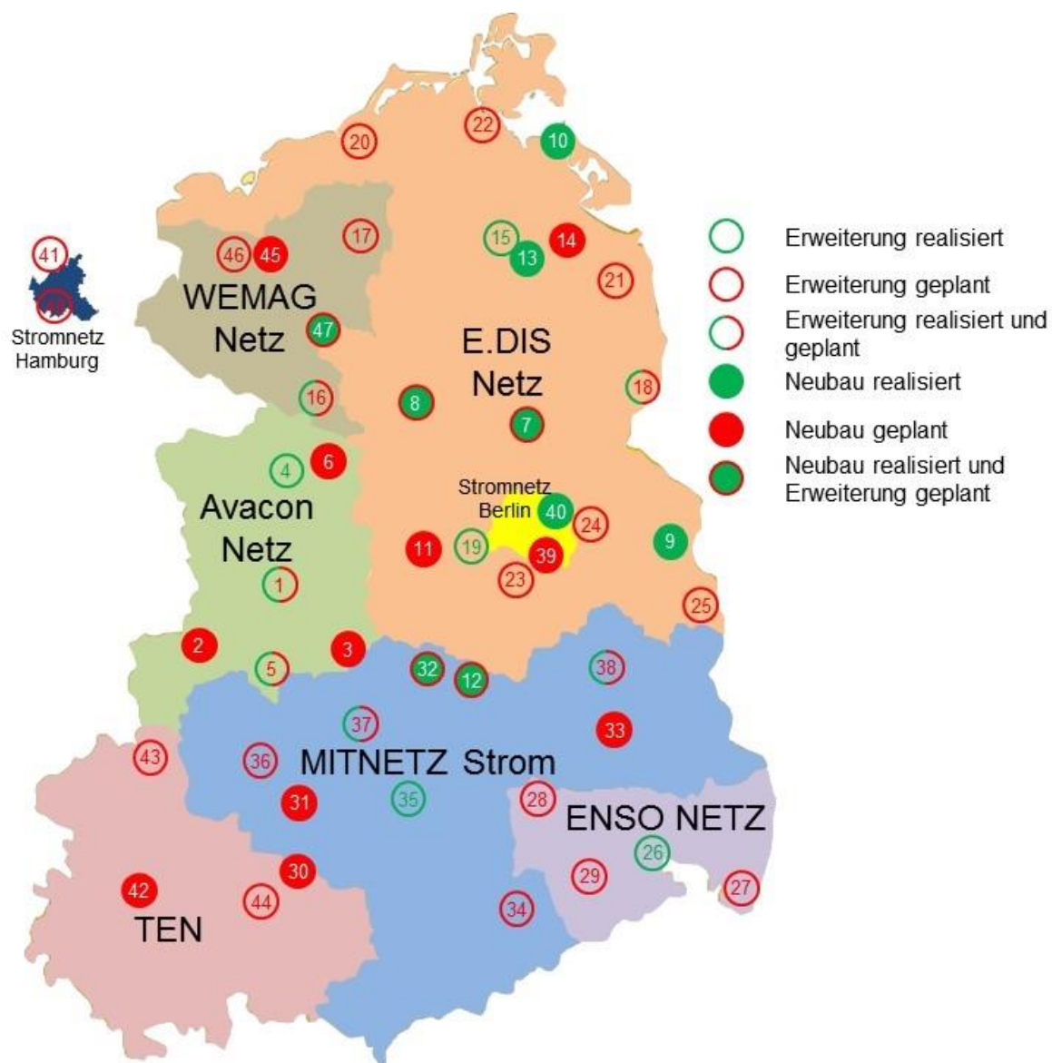
Abbildung 10: Darstellung der Ausbaumaßnahmen an Übergabepunkten zum Höchstspannungsnetz
