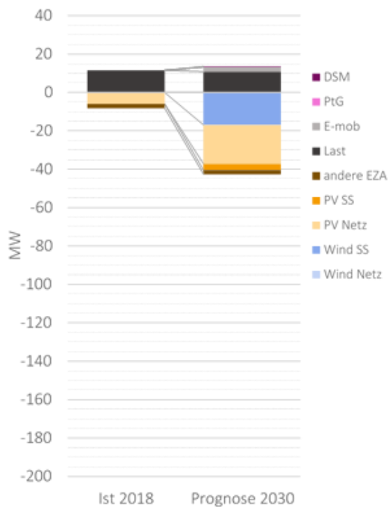
Leistungen im Lastfall Schwachlast/ starke Erzeugung
