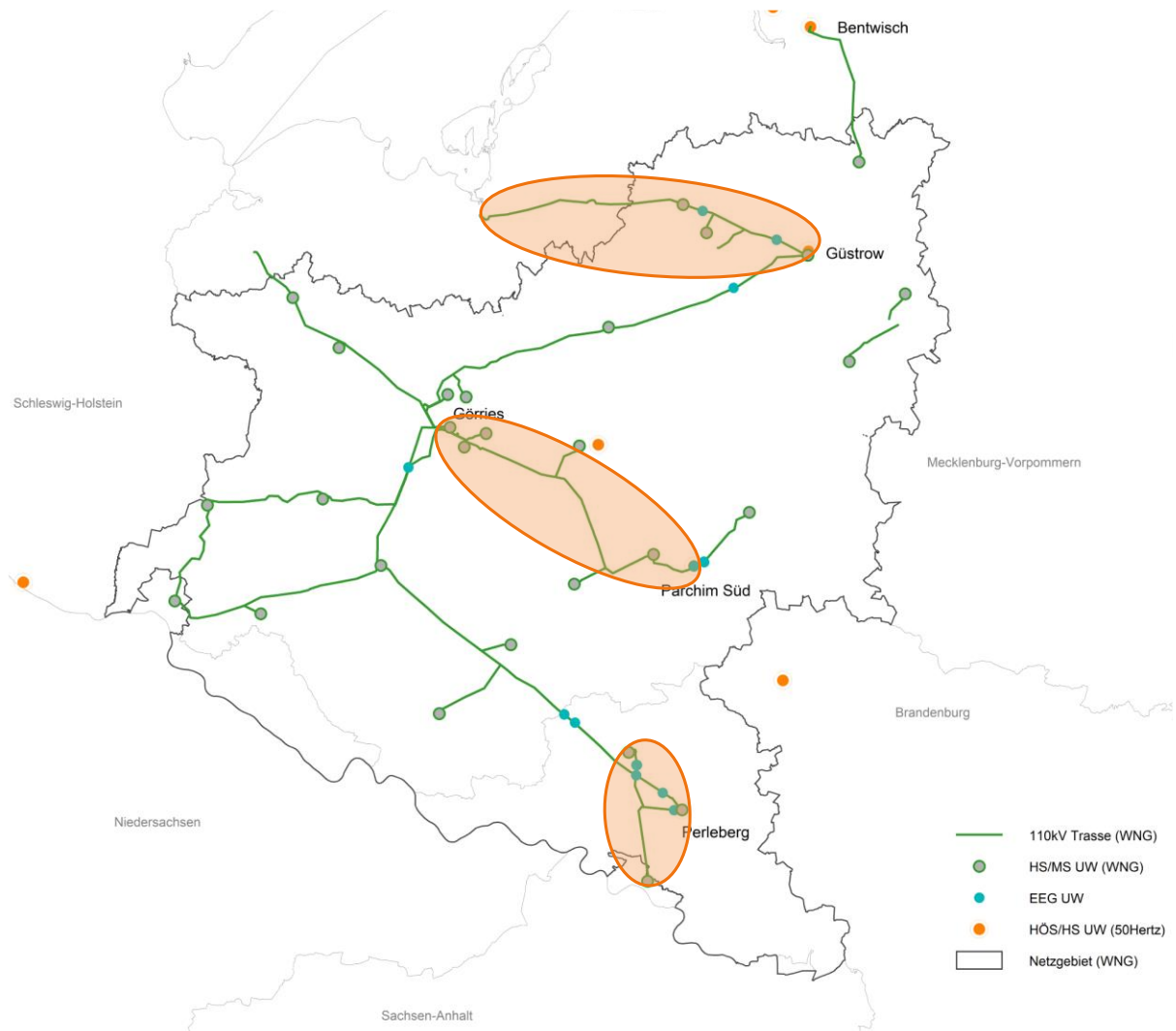
Abbildung 9: Engpässe im Hochspannungsnetz der WEMAG Netz
