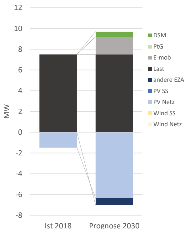
Leistungen im Lastfall Schwachlast/ starke Erzeugung
