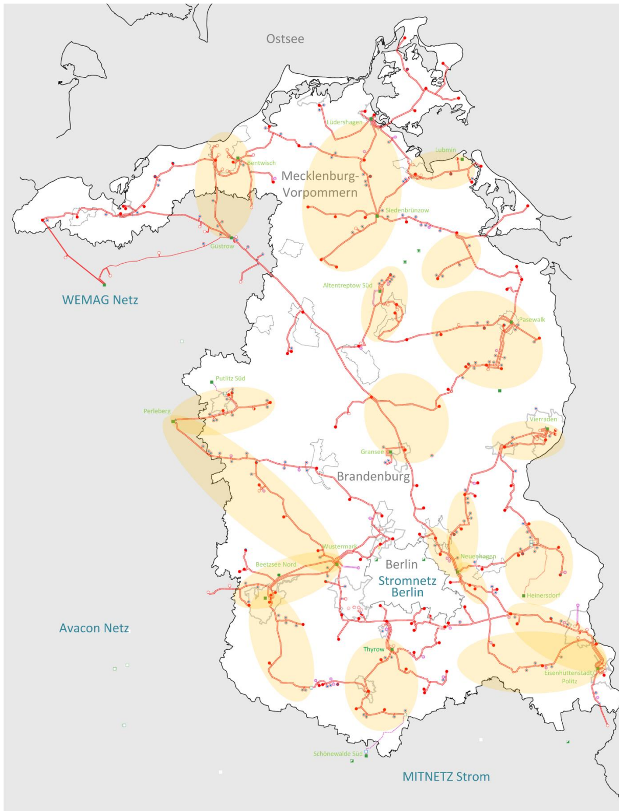
Abbildung 5: Engpässe im Hochspannungsnetz der E.DIS Netz
