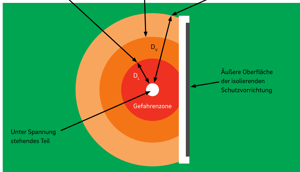
Bild 18: Gefahrenzone und Schutzabstände
