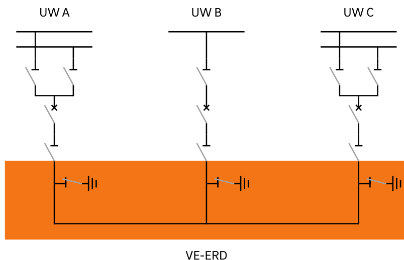
Bild 4: VE-ERD Hochspannung
