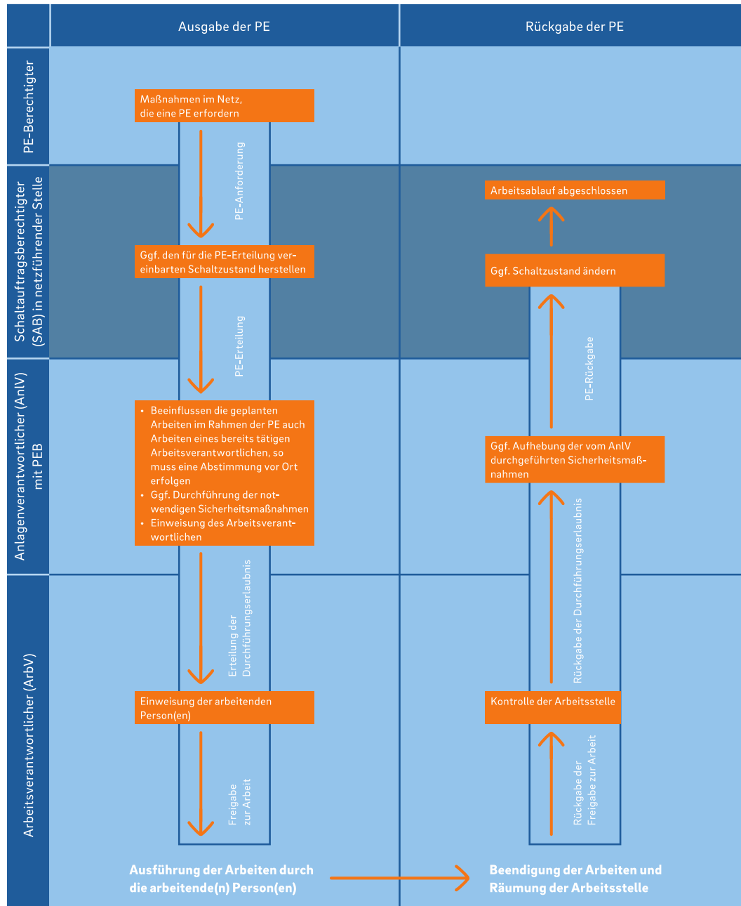
Bild 31: Arbeiten mit PE-Erteilung innerhalb von abgeschlossenen elektrischen Betriebsstätten
