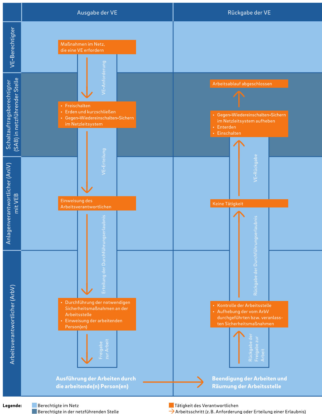
Bild 23: Arbeiten mit VE-ERD-Erteilung sowie Durchführung von Sicherheitsmaßnahmen durch den Arbeitsverantwortlichen
