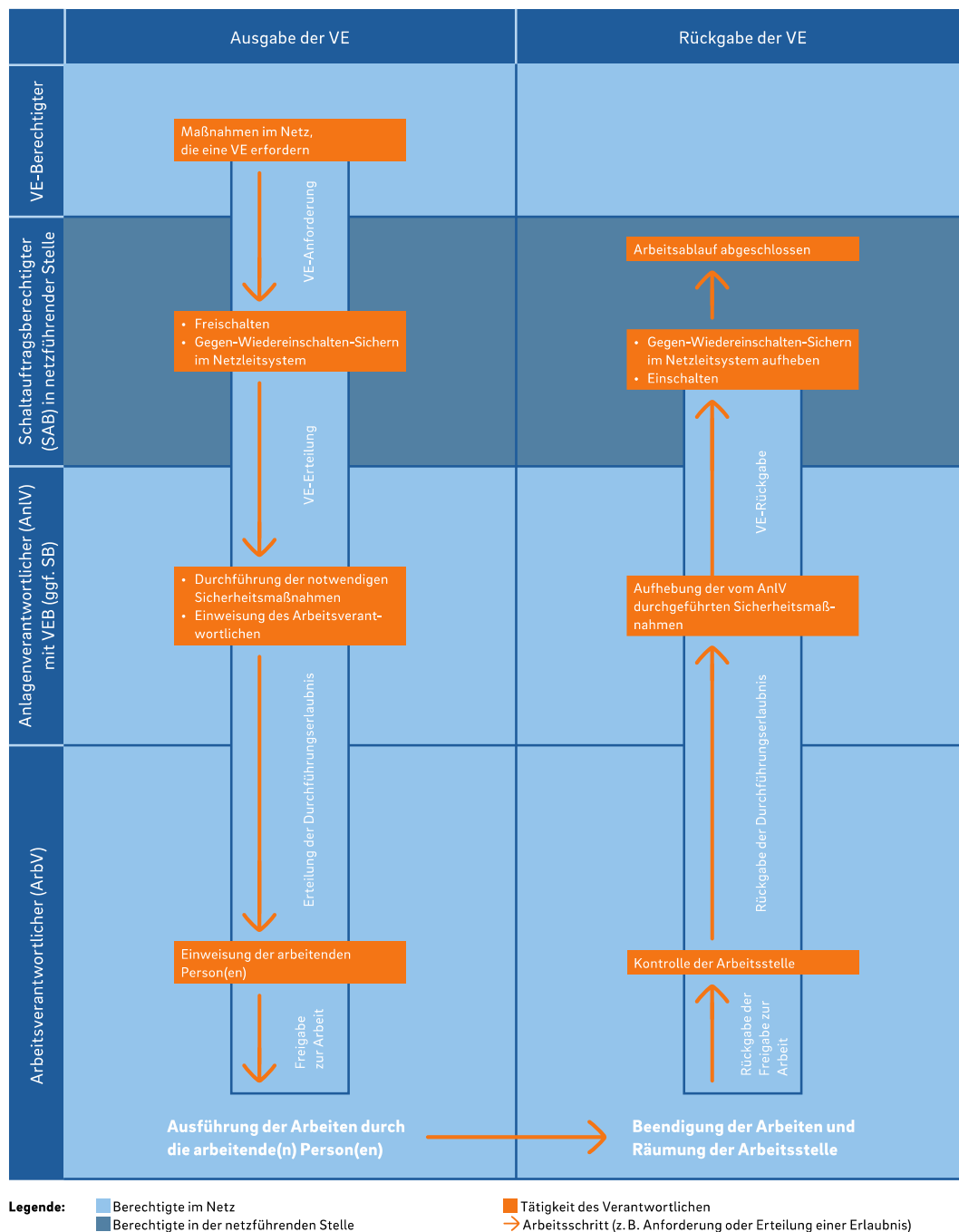
Bild 24: Arbeiten mit VE-FREI-Erteilung sowie Durchführung von Sicherheitsmaßnahmen durch den Anlagenverantwortlichen
