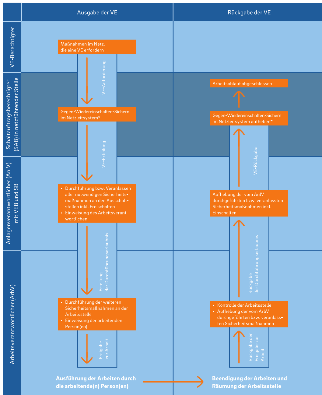
Bild 26: Arbeiten mit VE-EIN-Erteilung sowie Durchführung von Sicherheitsmaßnahmen durch den Anlagen- und Arbeitsverantwortlichen
