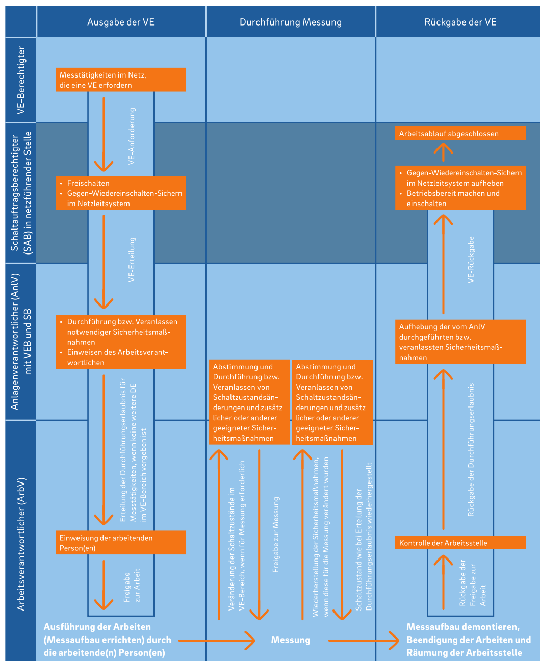
Bild 29: Messtätigkeiten mit VE-FREI sowie Durchführung von Sicherheitsmaßnahmen durch den Anlagenverantwortlichen
