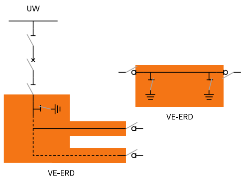
Bild 5: VE-ERD Mittelspannung
