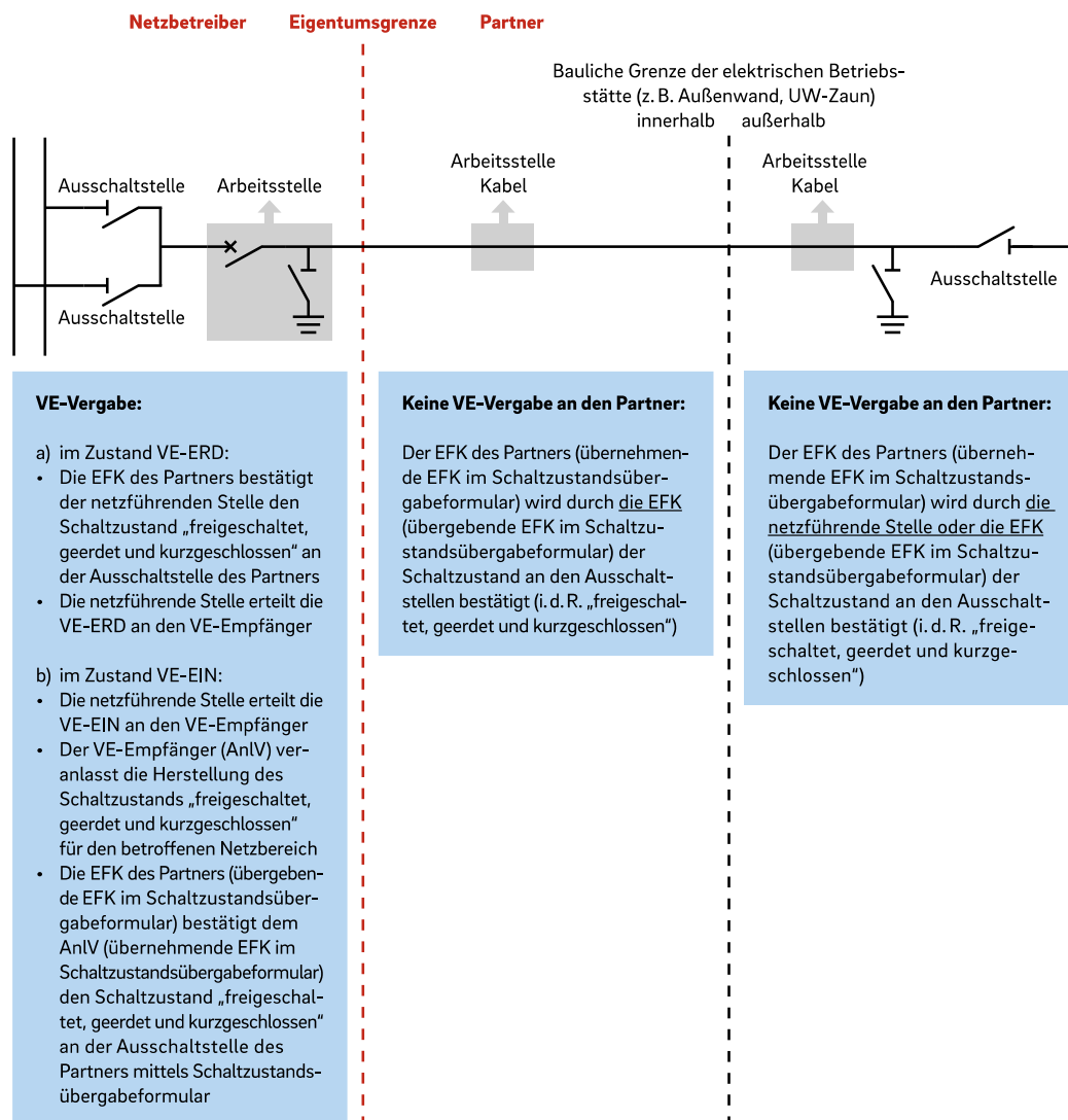
Bild 16: Austausch des Schaltzustands mit der EFK eines MS-Kunden
