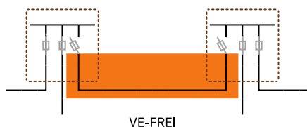
Bild 10: VE-FREI Niederspannung
