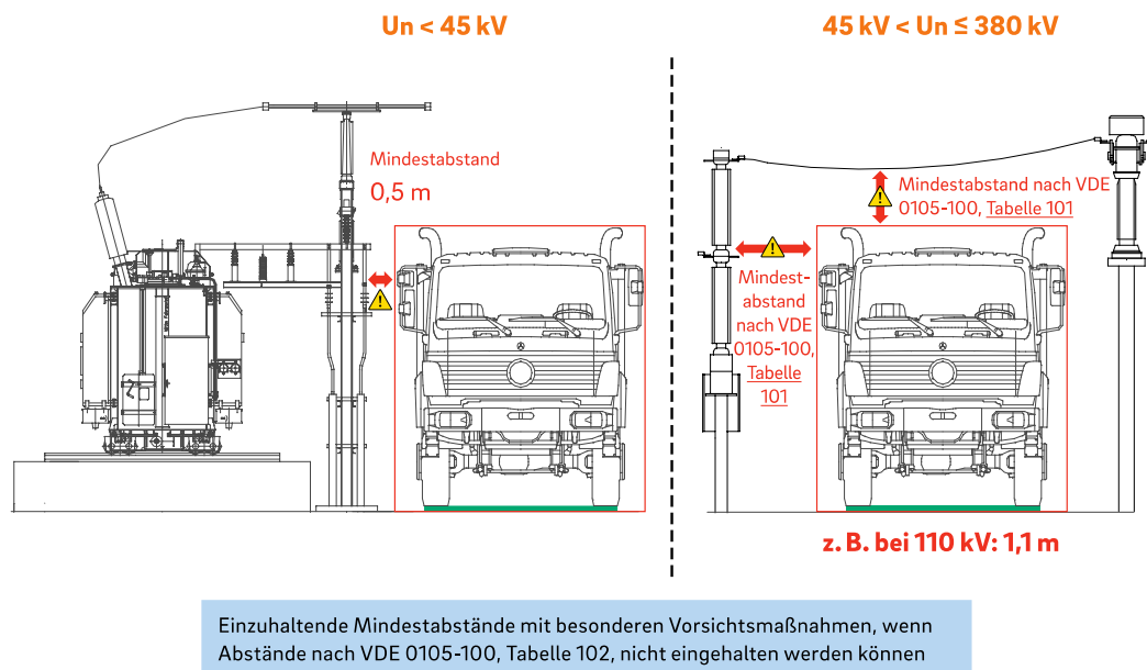
Bild 19: Fahrzeug-Schutzabstände
