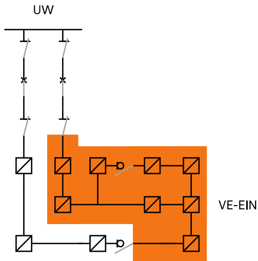
Bild 11: VE-EIN Mittelspannung
