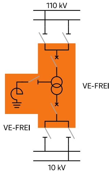
Bild 8: VE-FREI Transformator
