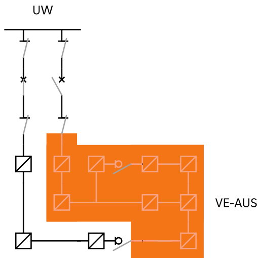
Bild 13: VE-AUS Mittelspannung
