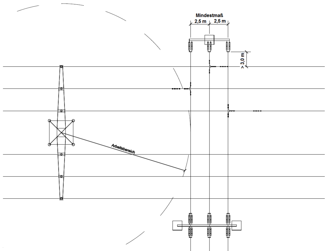
Abb. 4: Draufsicht
