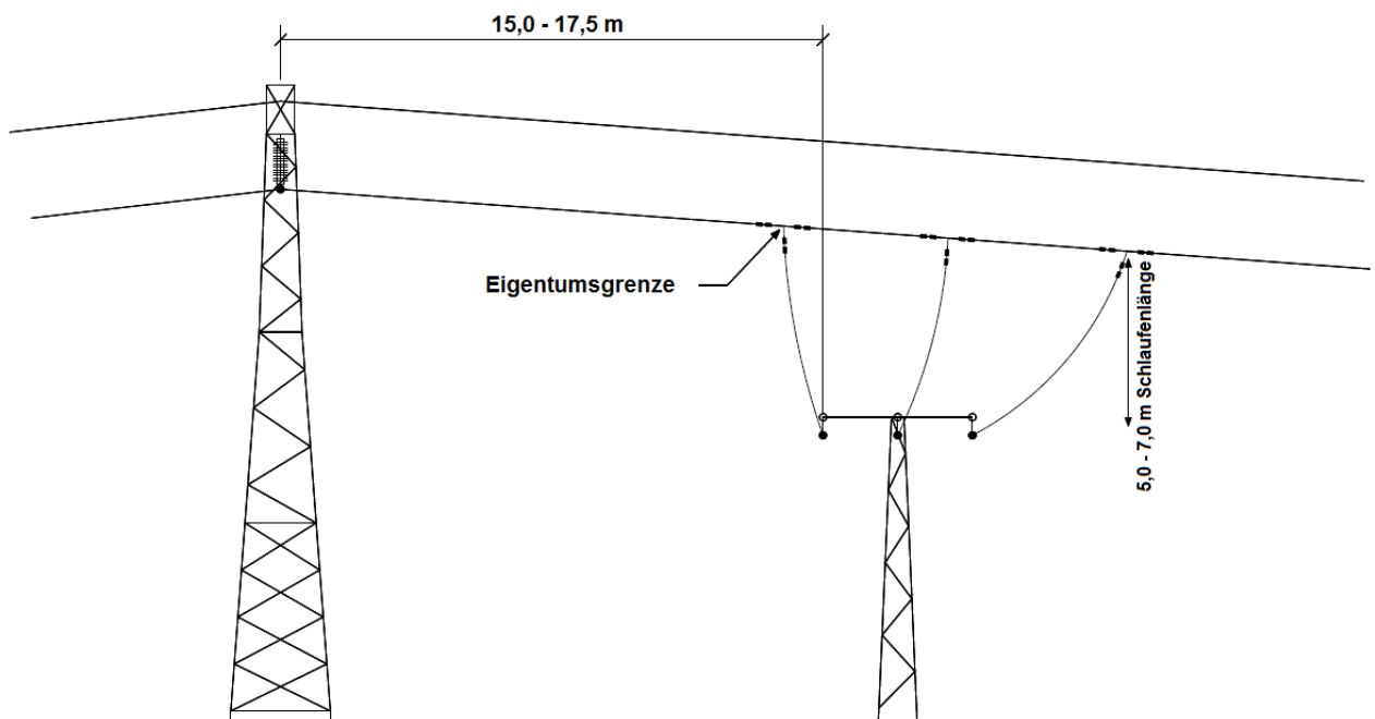
Abb. 3: Sicht quer zur Leitungsrichtung
