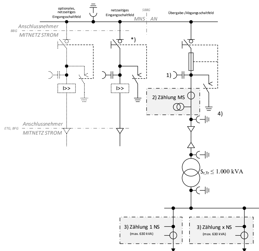
Abb. 23: (ehemals D1a): \leq 20 -kV-Anbindung mit einem Abgangsfeld; Transformator \leq 1 MVA (z.B. 630 kVA)
