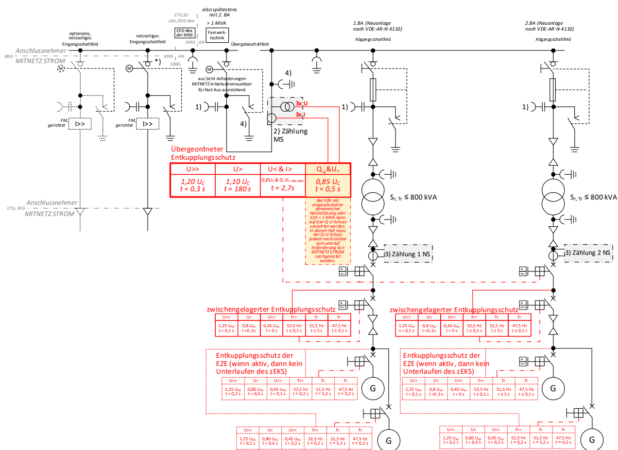
Abb. 32: (ehemals D4e): \leq 20 -kV-Anbindung von zwei Bauabschnitten einer PV-Anlage mit je 750 kVA (spätestens ab 2.BA mit FWT, in diesem Fall im 1.BA mit FRE)
