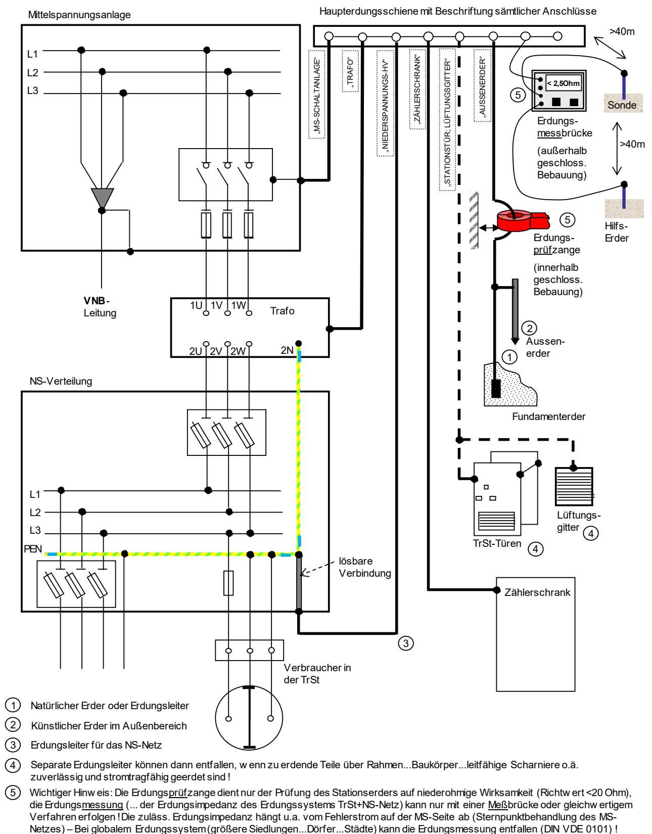
Abb. 8: Gemeinsame Mittel- und Niederspannungs-Erdsungsanlage in einer Übergabestation
