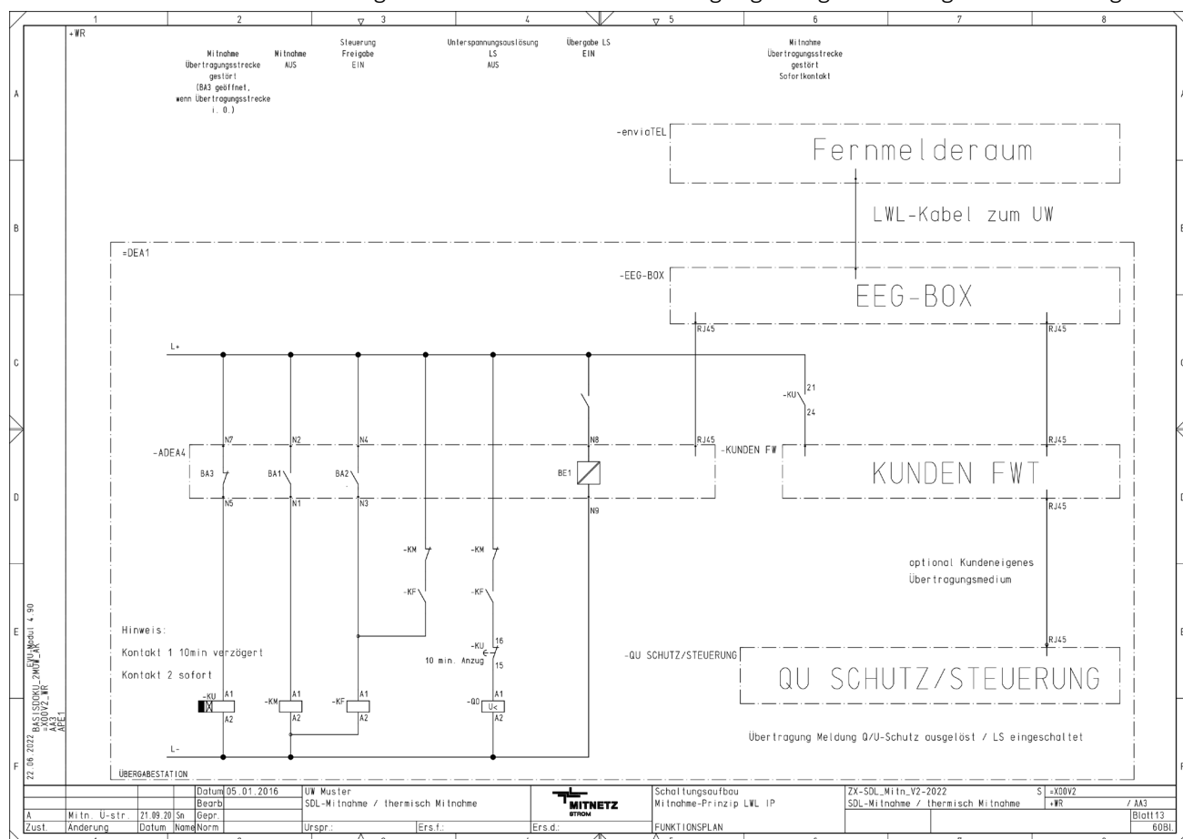
Abb. 51: Schaltungsaufbau der LVL-Kabelverbindung zwischen der Übergabestation und dem MITNETZ STROM-Umspannwerk (Standardfall)
