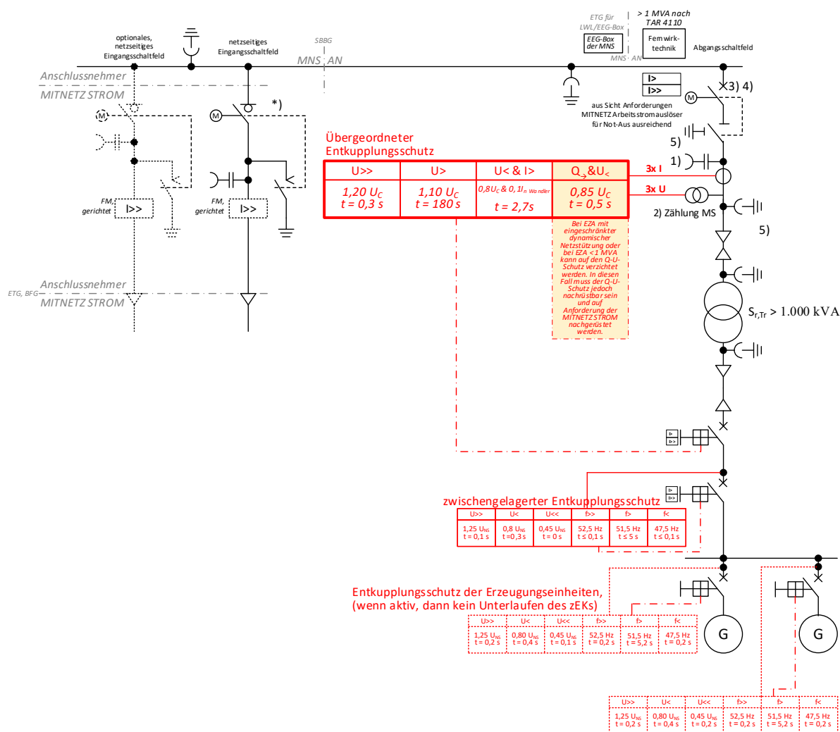
Abb. 31: (ehemals D4d): ≤ 20-kV- Anbindung einer Erzeugungsanlage &gt; 1 MVA
