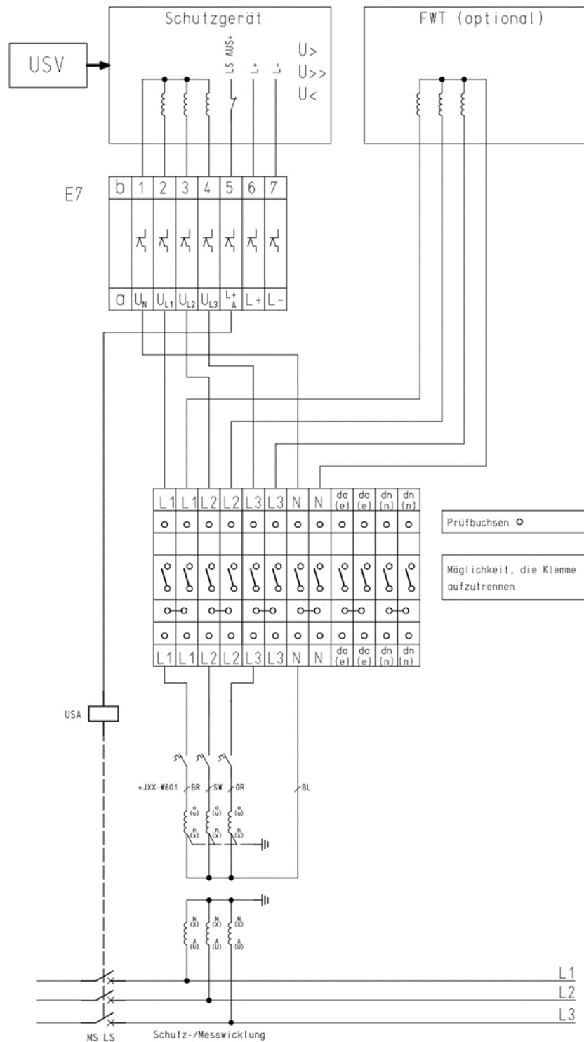
Abb. 48: Wandlerverdrahtung Anbindung übergeordneter Entkupplungsschutz / Fernwirkgerät
