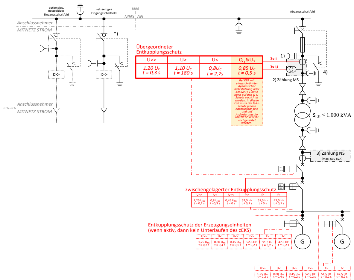
Abb. 30: (ehemals D4c): \leq 20 -kV-Anbindung einer Erzeugungsanlage \leq 1 MVA
