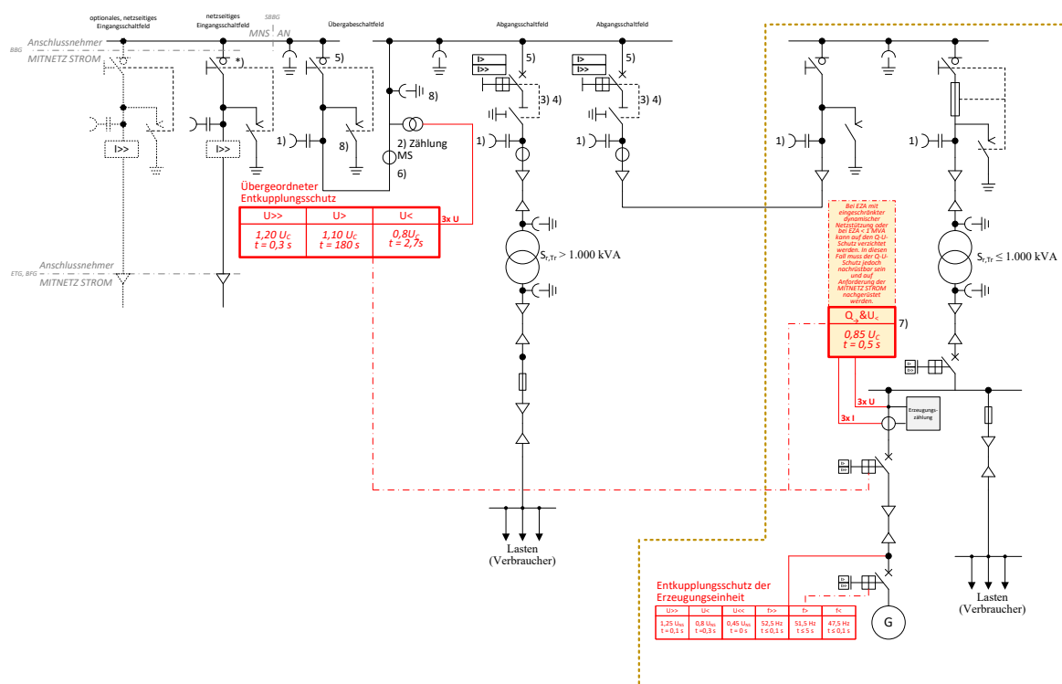
Abb. 35: (ehemals D5c): \leq 20 -kV-Anbindung einer Mischanlage mit nachgelagerter Station
