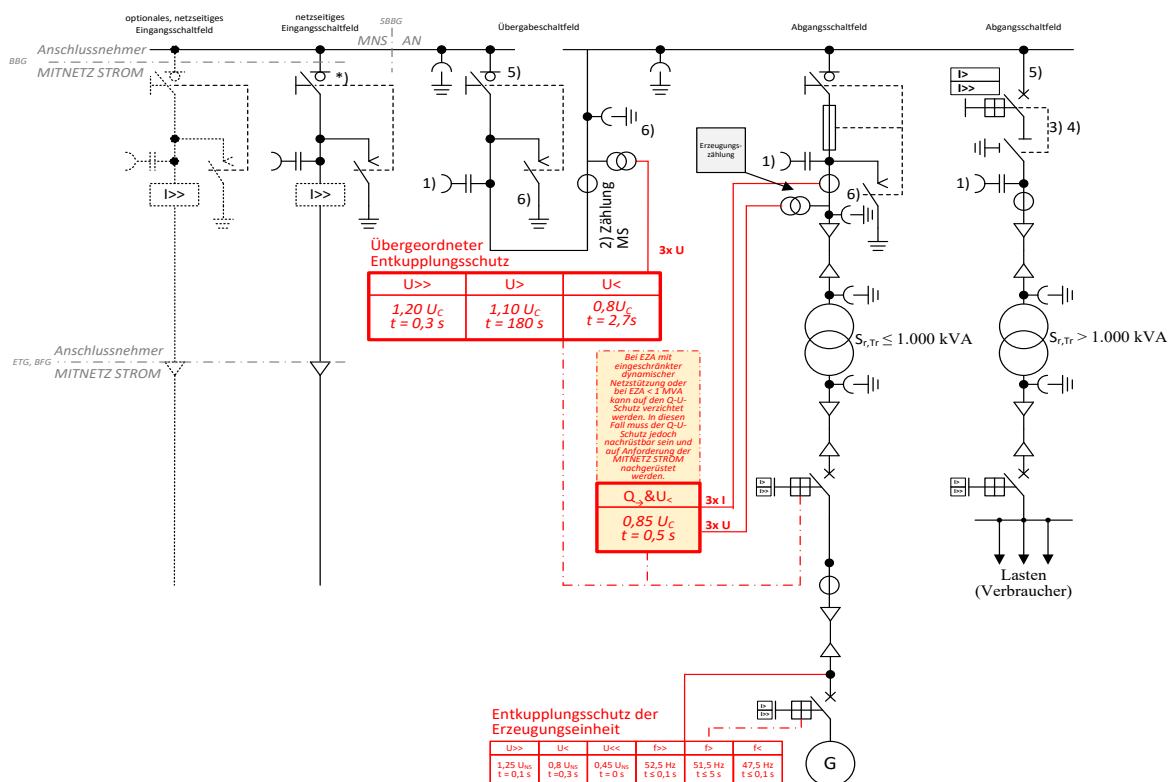
Abb. 34: (ehemals D5b): \leq 20 -kV-Anbindung einer Mischanlage über je einen Transformator für Bezug und Einspeisung
