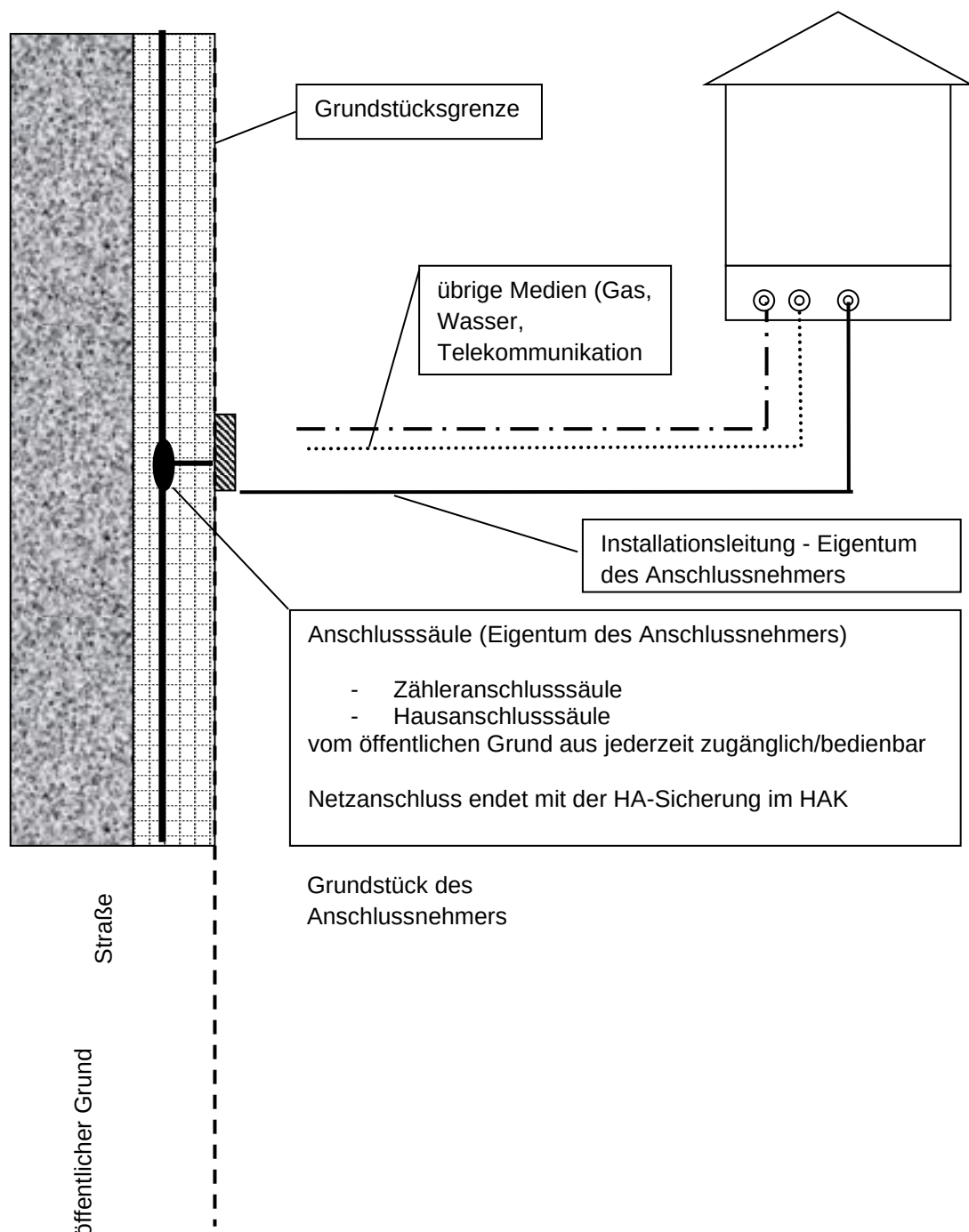
Abb. 5: Beispiel für Außenanschlusstechnik mit Anschlussäule
