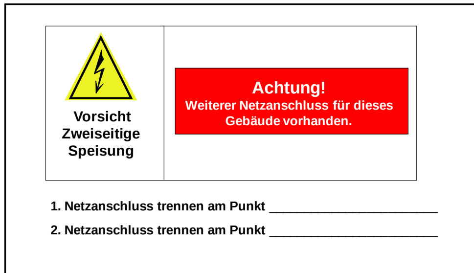
Abb. 12: Hinweisschild „Achtung! Weiterer Netzanschluss für dieses Gebäude vorhanden.“
