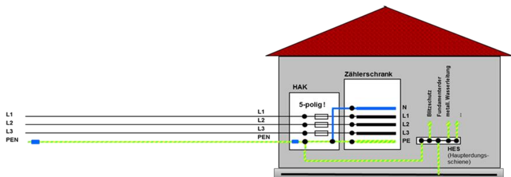
Abb. 18: Anschlussvariante bei MITNETZ STROM zur Innenanschlusstechnik (beispielhafte Darstellung)
