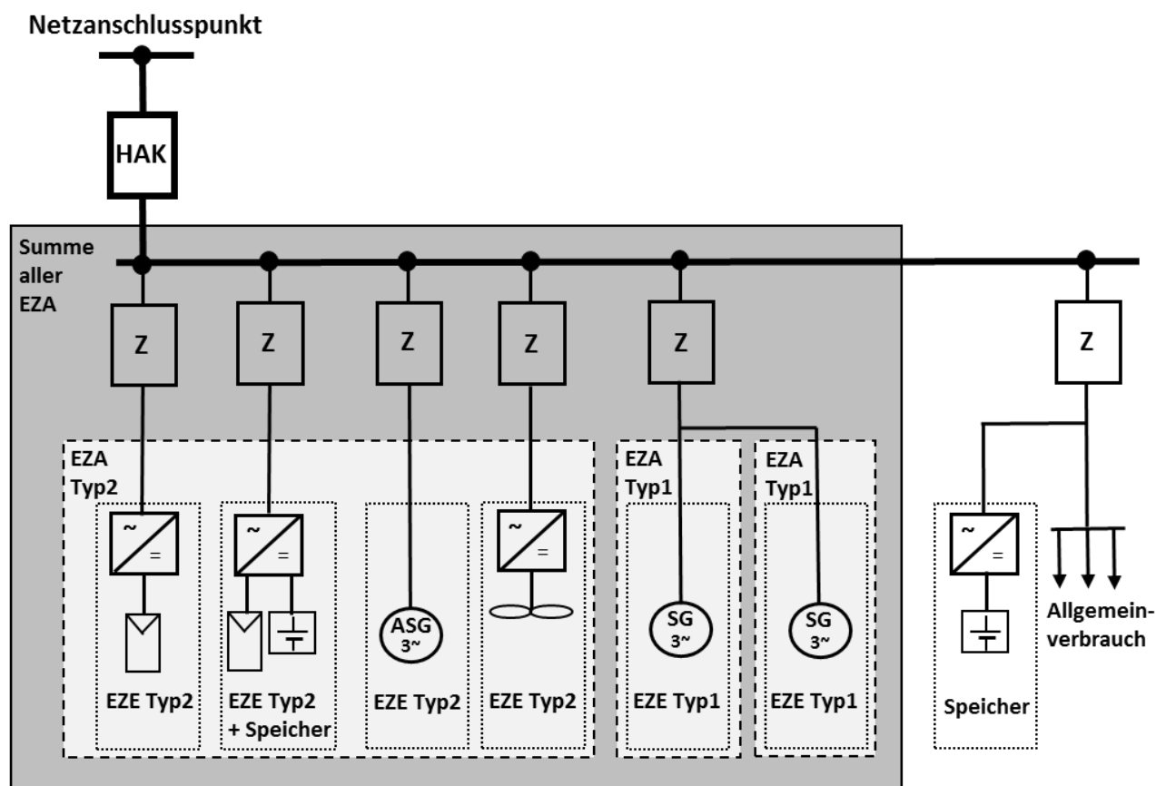
Abb. 9: Erläuterung der Begriffe Erzeugungseinheit (EZE) und Erzeugungsanlage (EZA)
