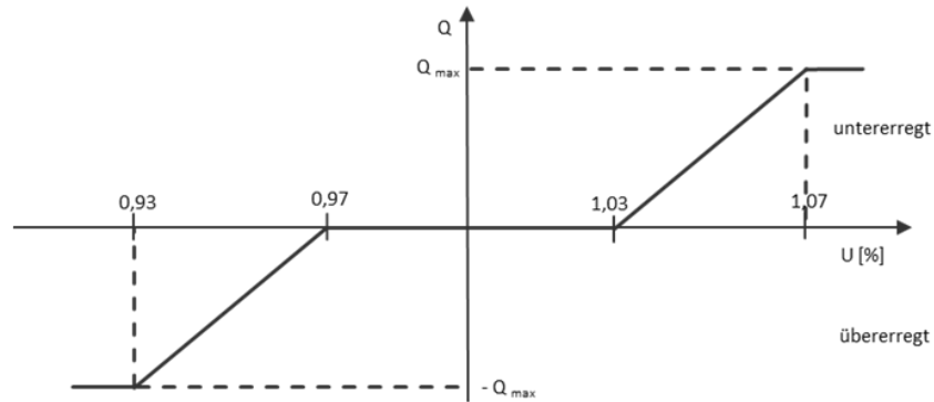
Abb. 15: Standard - Kennlinie für Q(U)
