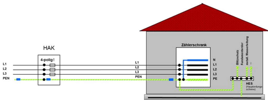
Abb. 17: Anschlussvariante bei MITNETZ STROM zur Außenanschlusstechnik (beispielhafte Darstellung)
