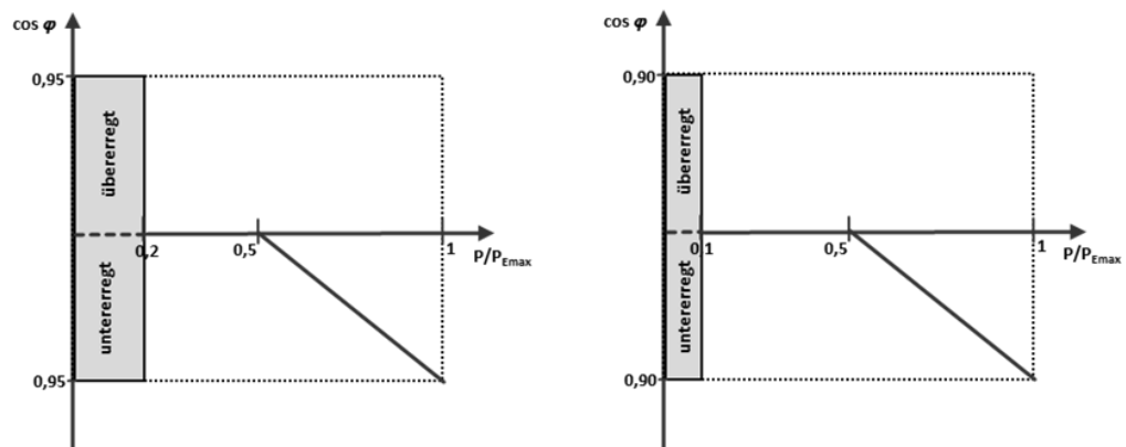
Abb. 16: Standard - Kennlinie für \cos \varphi (P)
