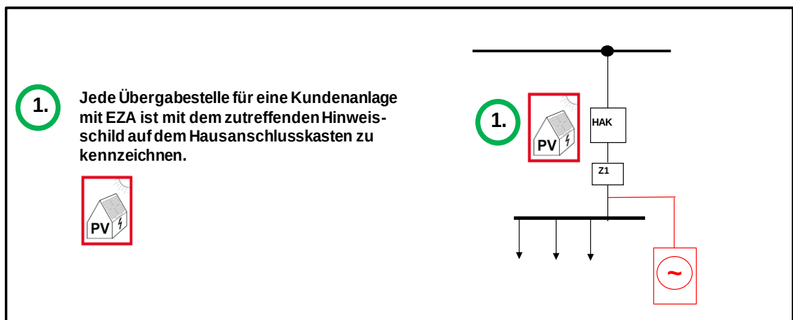
Abb. 13: : Kennzeichnung der Kundenanlage mit Hinweisschildern „Erzeugungsanlage“ (beispielhaft)
