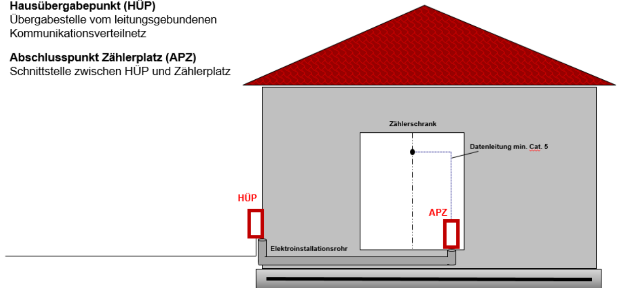
Abb. 8: Anbindung von Kommunikationseinrichtungen (beispielhaft)
