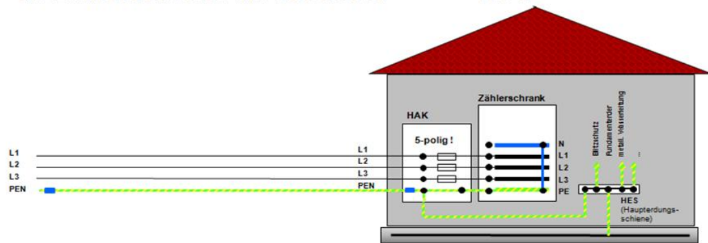
Abb. 19: Anschlussvariante bei MITNETZ STROM zur Innenanschlusstechnik (beispielhafte Darstellung)
